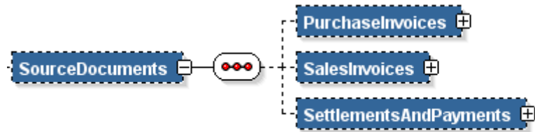
Paveikslėlis Nr. 12. i.SAF XSD - SourceDocuments
