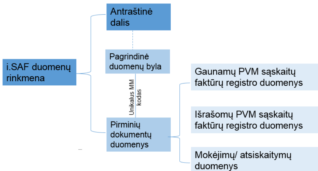
Paveikslėlis Nr. 2. i.SAF duomenų rinkmenos apibendrinta struktūra
