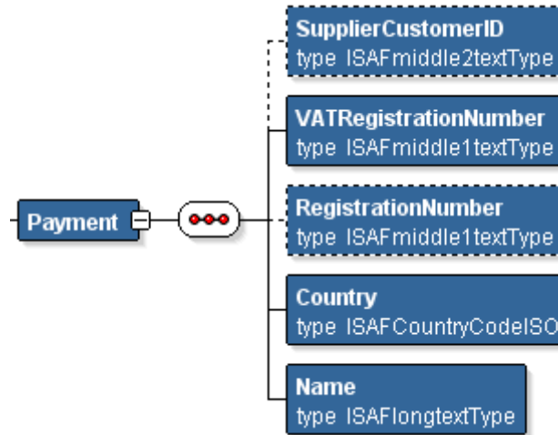
Paveikslėlis Nr. 22. i.SAF XSD - Payment
