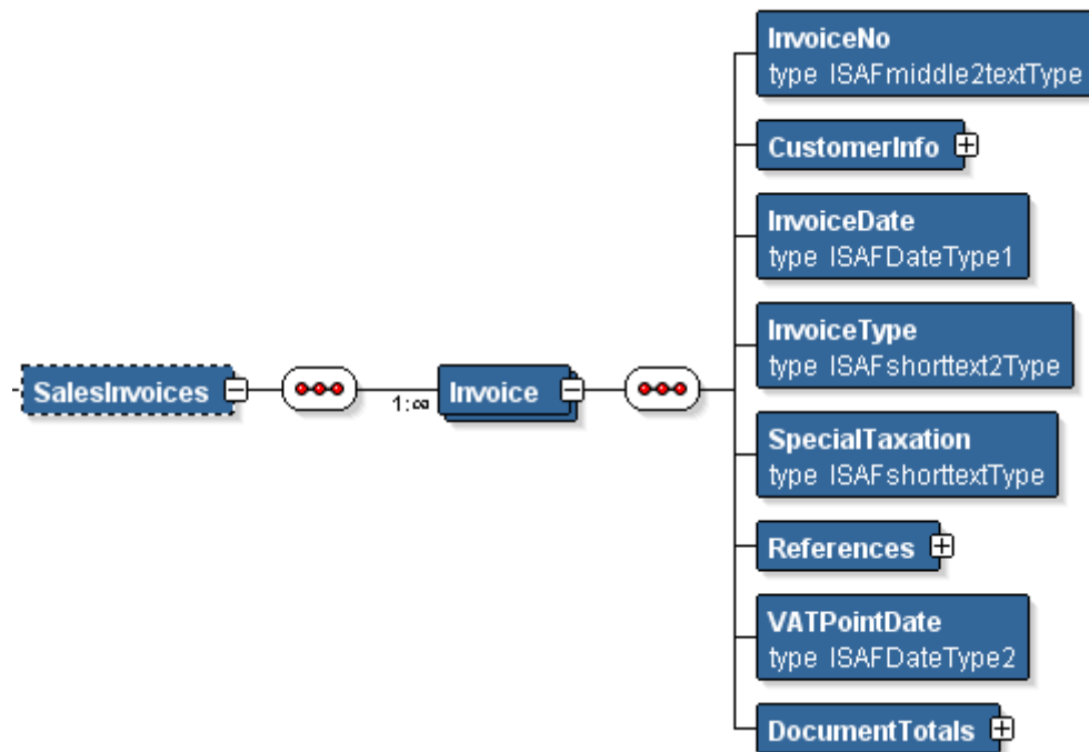
Paveikslėlis Nr. 17. i.SAF XSD - Invoice (SalesInvoices)
