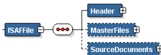
Paveikslēlis Nr. 5. i.SAF XSD -ISAFFile
