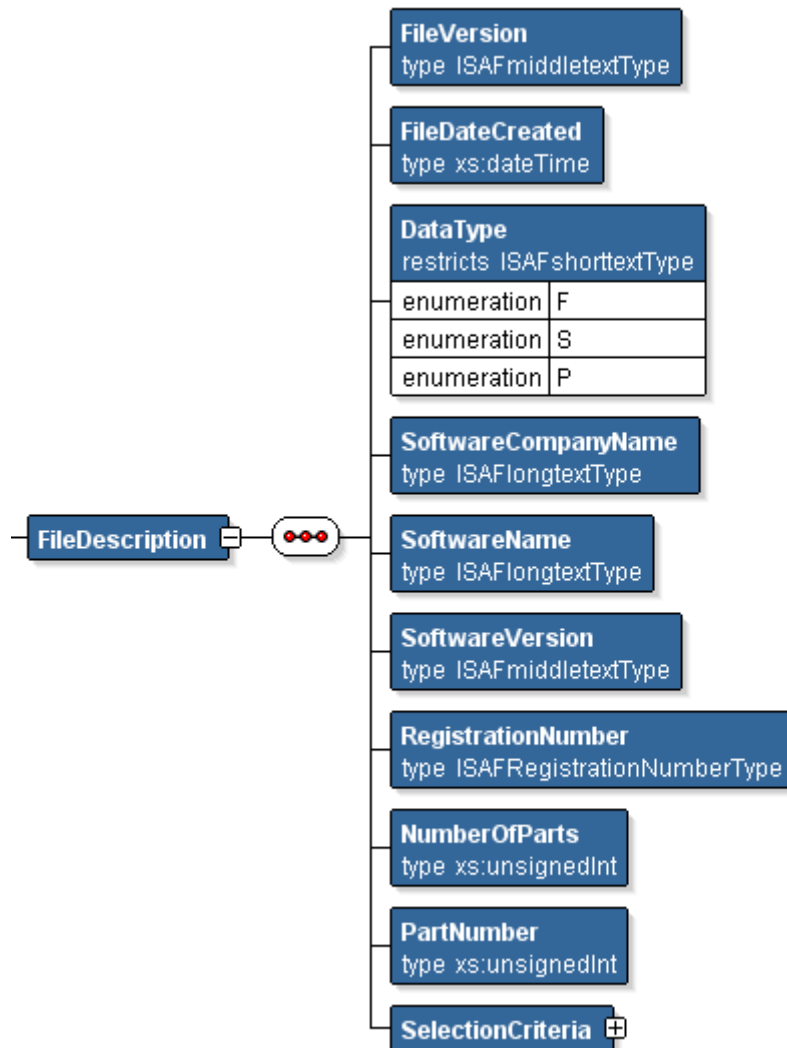
Paveikslėlis Nr. 7. i.SAF XSD - FileDescription
