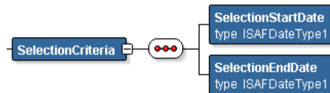
Paveikslėlis Nr. 8. i.SAF XSD - SelectionCriteria
