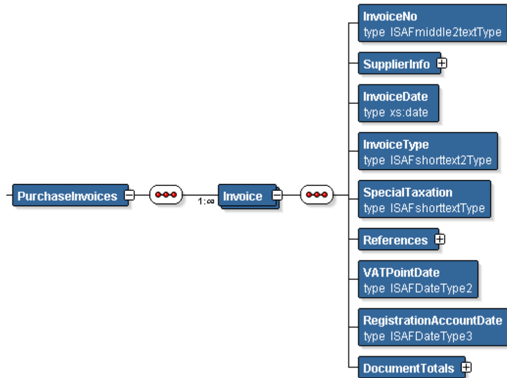
Paveikslėlis Nr. 13. i.SAF XSD - Invoice (PurchaseInvoices)
