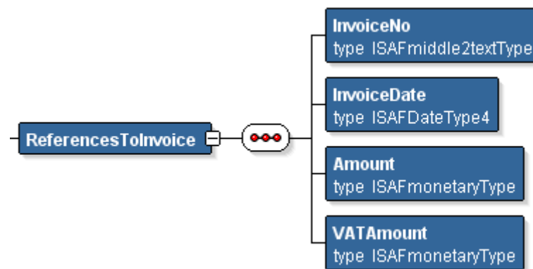
Paveikslėlis Nr. 23. i.SAF XSD - ReferencesToInvoice
