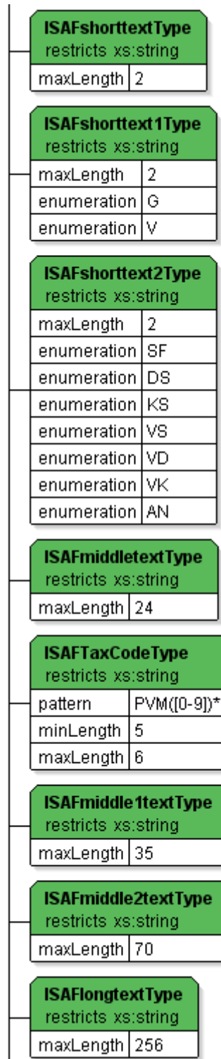
Paveikslėlis Nr. 24. Paprastieji tipai (1)
