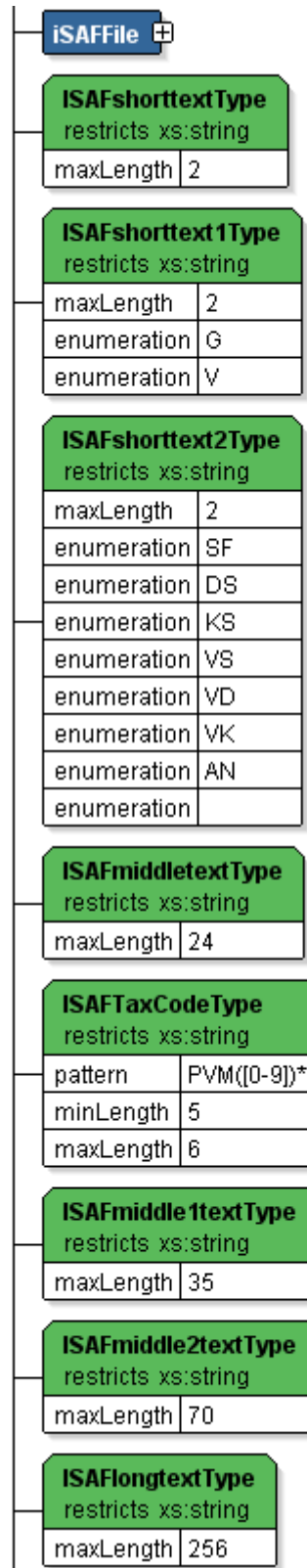
Paveikslėlis Nr. 3. i.SAF XSD - i.SAF bendra struktūra(1)
