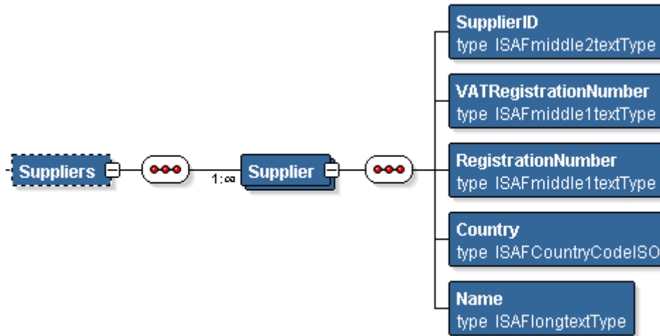
Paveikslėlis Nr. 11. i.SAF XSD - Supplier (Suppliers)
