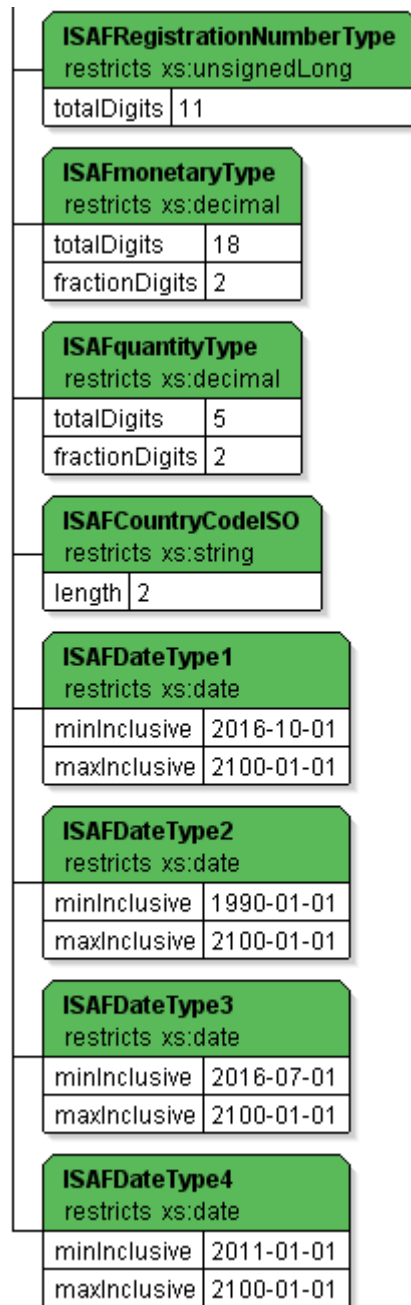
Paveikslēlis Nr. 4. i.SAF XSD - i.SAF bendra struktūra(2)
