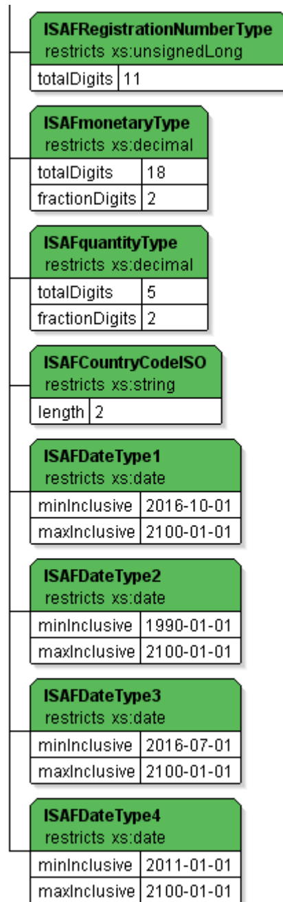
Paveikslėlis Nr. 25. Paprastieji tipai (2)
