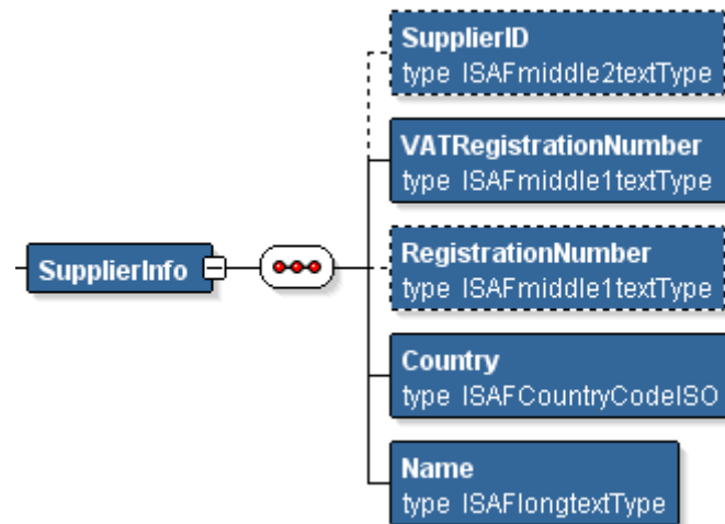
Paveikslėlis Nr. 14. i.SAF XSD - SupplierInfo
