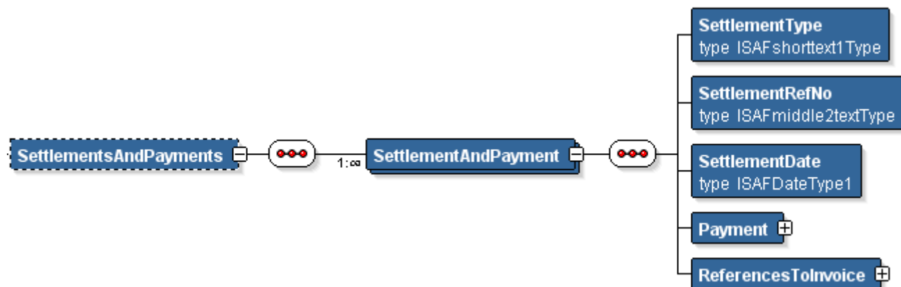
Paveikslėlis Nr. 21. i.SAF XSD - SettlementsAndPayment (SettlementsAndPayments)
