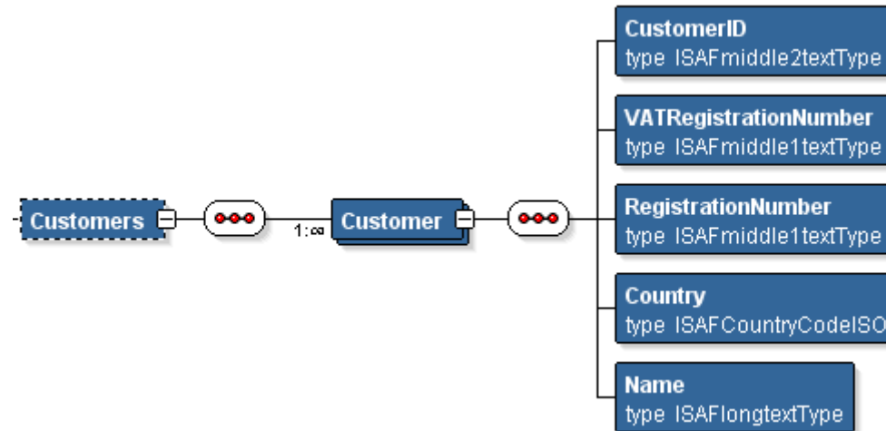
Paveikslėlis Nr. 10. i.SAF XSD - Customer (Customers)
