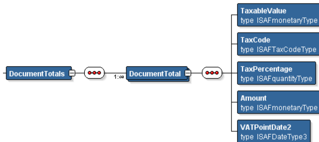
Paveikslėlis Nr. 20. i.SAF XSD - DocumentTotal (DocumentTotals)
