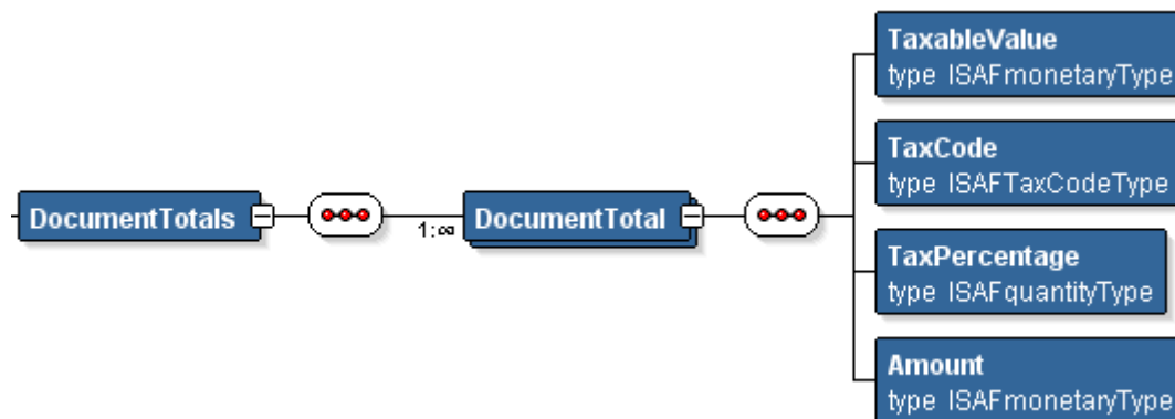
Paveikslėlis Nr. 16. i.SAF XSD - DocumentTotal ( DocumentTotals )
