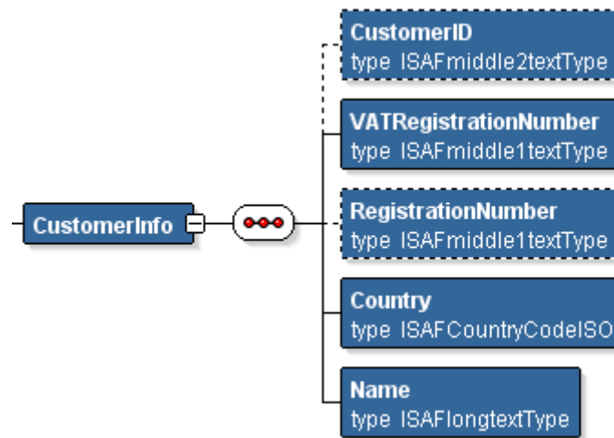
Paveikslėlis Nr. 18. i.SAF XSD - CustomerInfo
